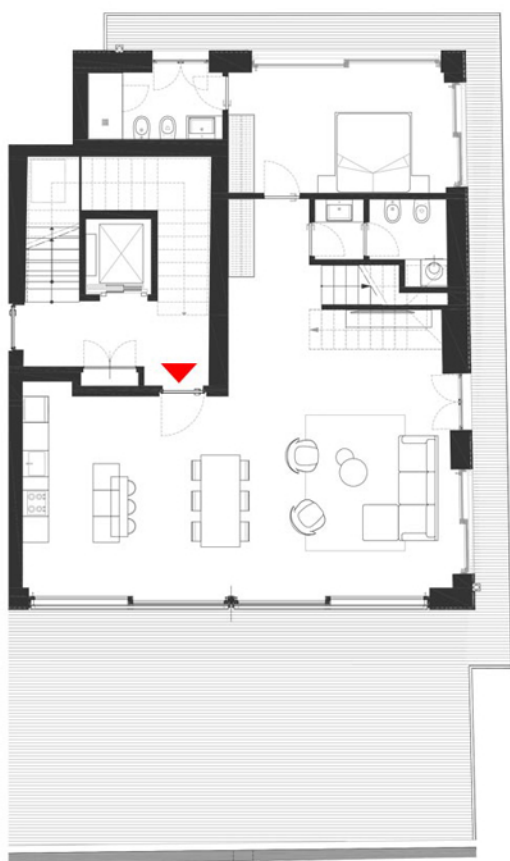
4° piano
